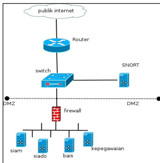
Gambar 2. Penempatan SNORT pada DMZ
