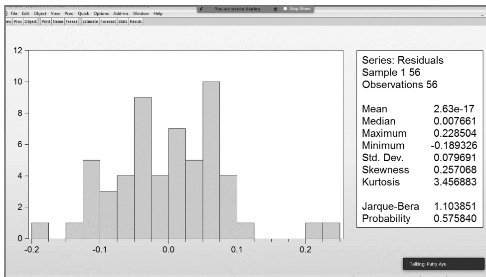
Gambar 1. Uji Normalitas
